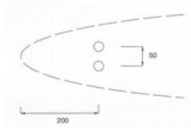
Aansluiting Blade H aan de achterzijde van de radiator.
